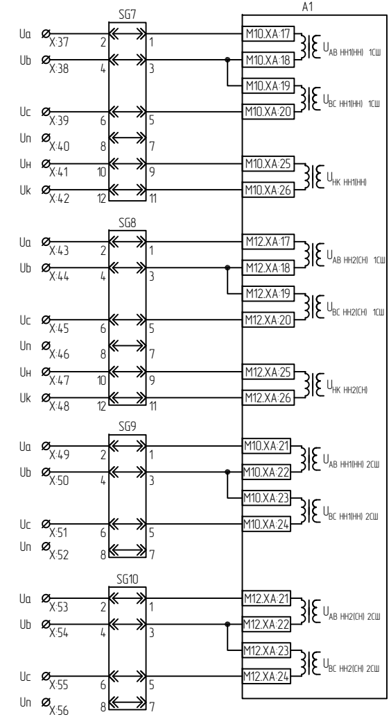
Цепи переменного и напряжения А1
